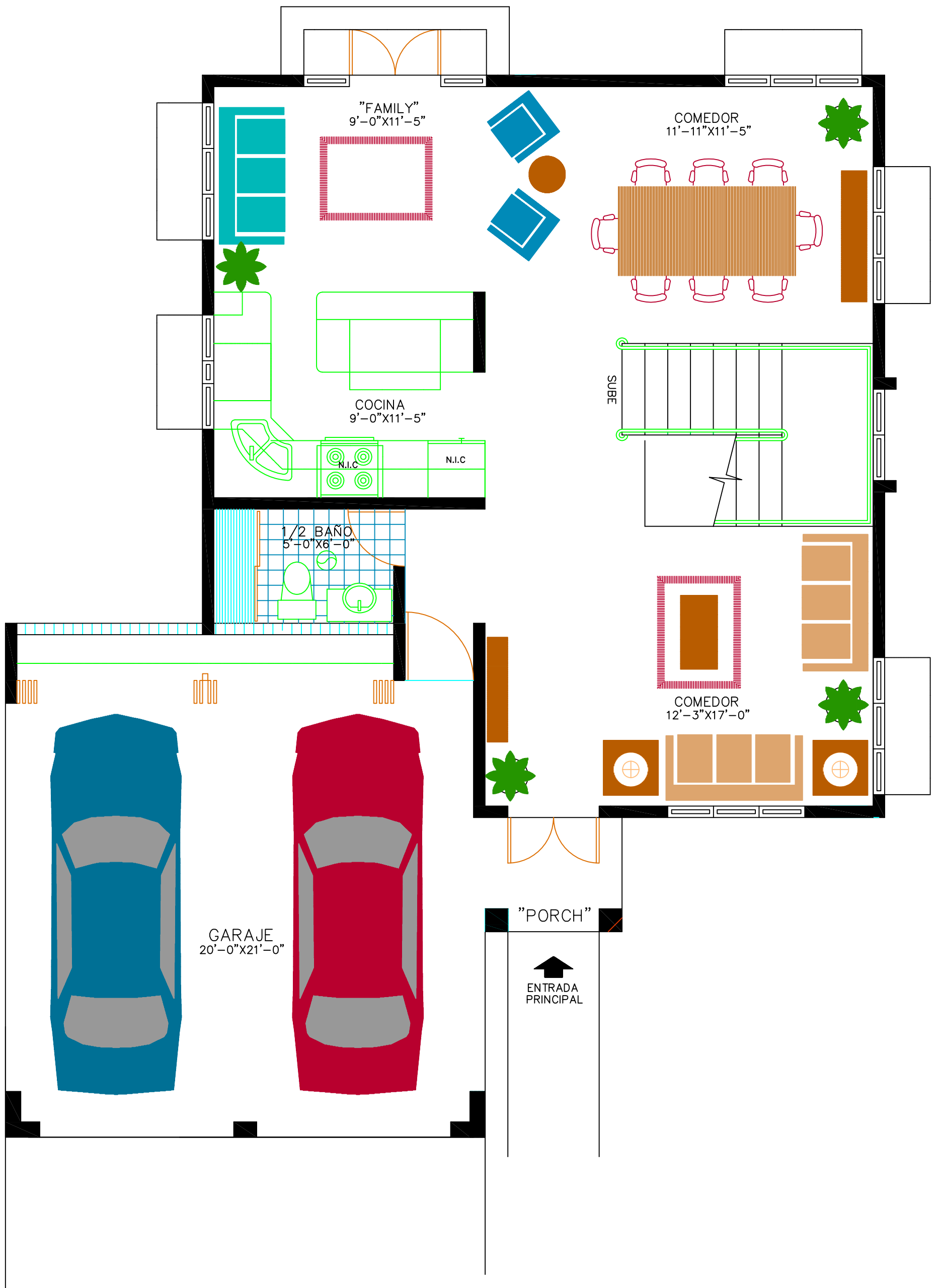
PRIMERA PLANTA DE PISO
